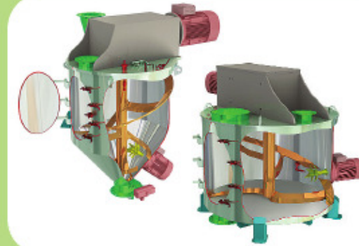
Κάθετα δοχεία ανάμιξης AMIXON.
